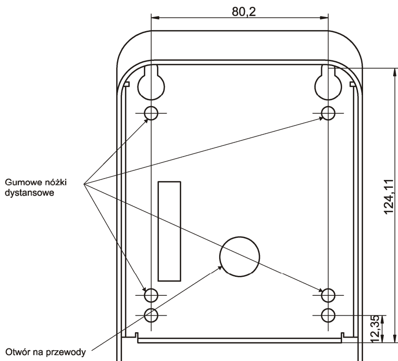
Rys.1 Widok wnętrza obudowy ME-9
